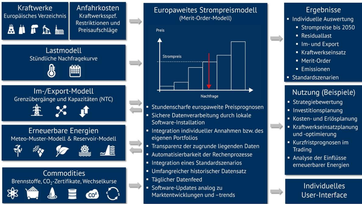
Abbildung 24: Funktionsschema Power2Sim
